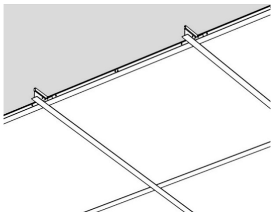
T-profiilile paigaldus
